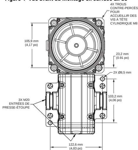
Figure 4 Vue avant du montage en surface Ex de
